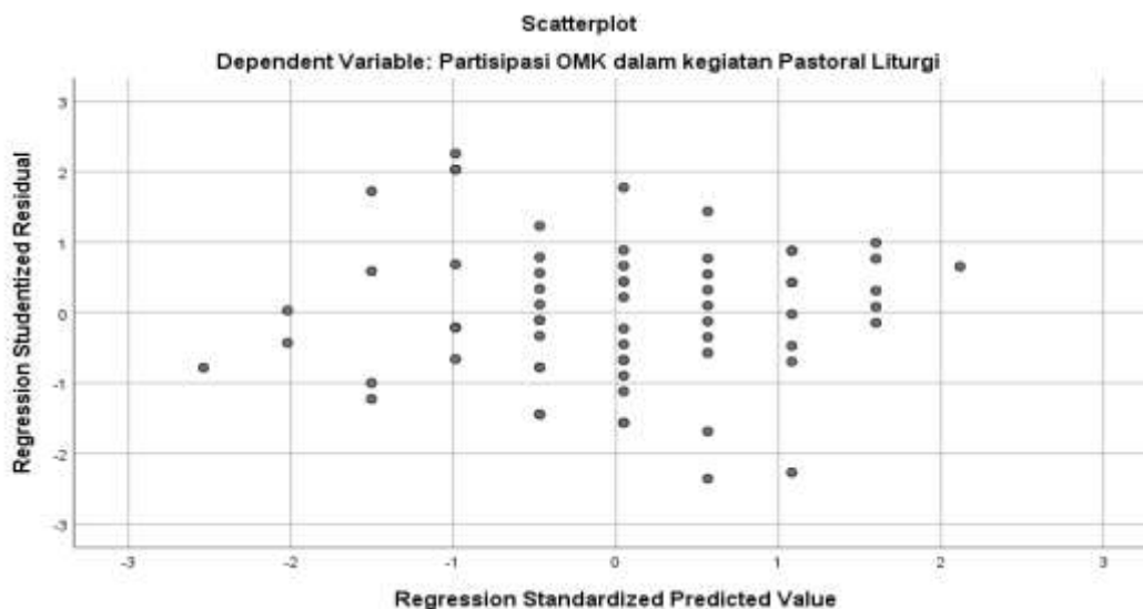
Gambar 10. Grafik scatter plot uji heteroskedastisitas
