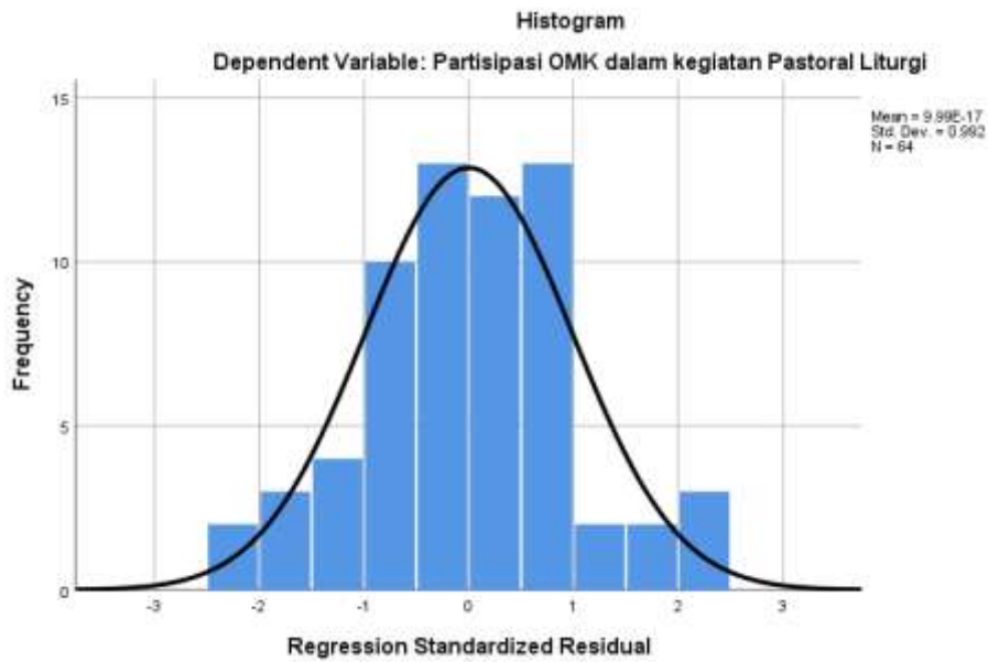
Gambar 9. Kurva hasil uji linearitas
